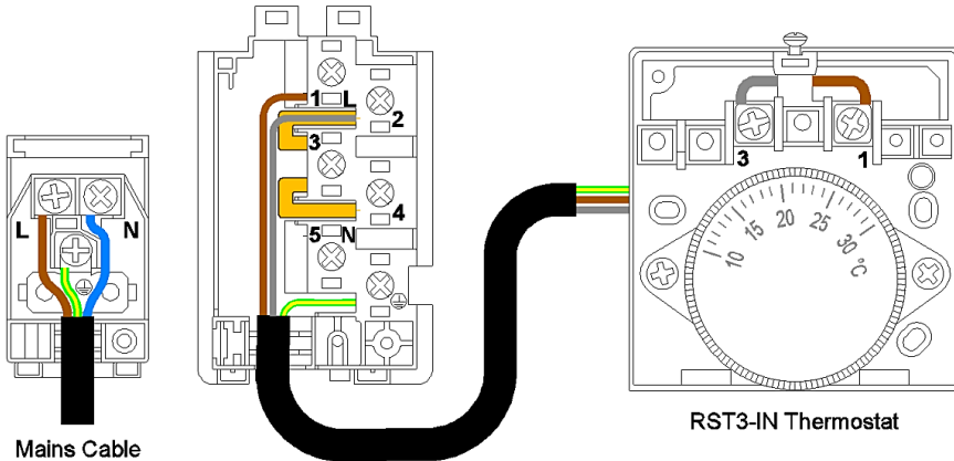
Mains Cable
